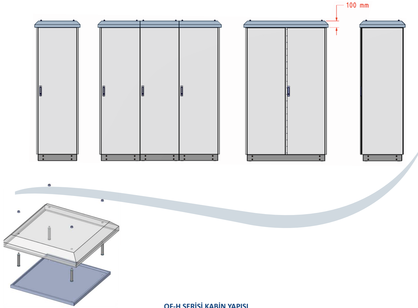
QF-H SERİSİ KABİN YAPISI
